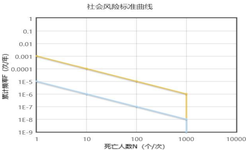
图 6.1-1 社会风险标准曲线图
