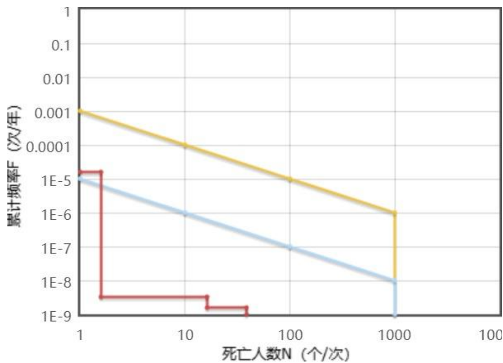
图 6.2-2 区域总体社会风险模拟图
