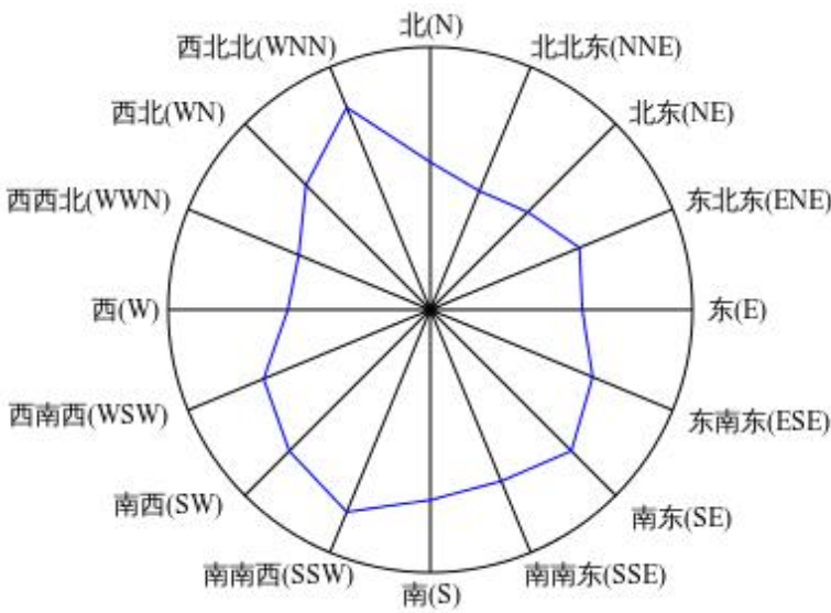
图 6.1-2 天津风向玫瑰图
