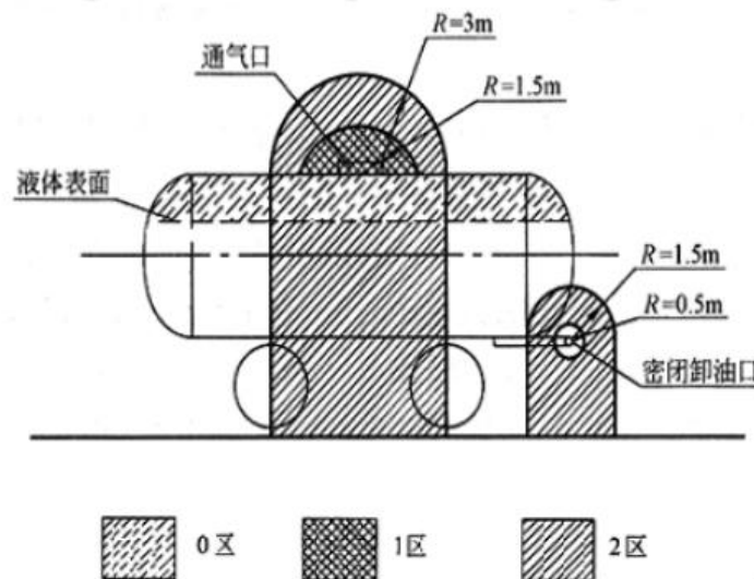
图 2.6-2 油罐车卸汽油时爆炸危险区域划分
