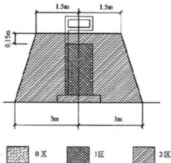
图 2.6-3 汽油加油机爆炸危险区域划分图
