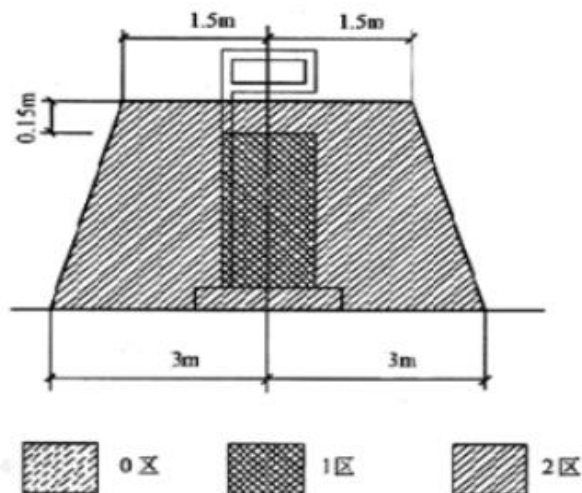
图 2.6-3 汽油加油机爆炸危险区域划分图
