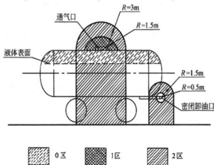
图 2.6-2 油罐车卸汽油时爆炸危险区域划分
